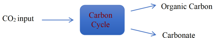
图 22 全球碳循环的简化图
