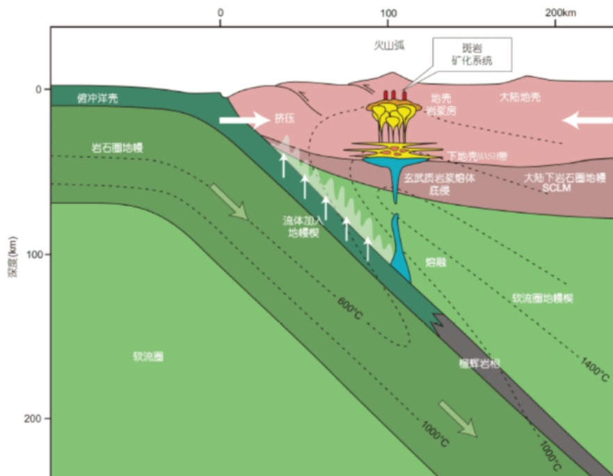
图 10 斑岩铜矿成矿模式
