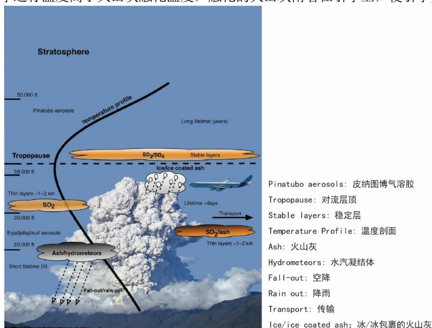
图21. 猛烈的火山喷发物在大气中的分布和对航空器的影响 (Prata & Rose, 2015)
