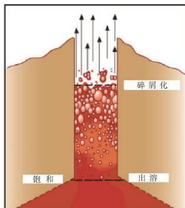
图16. 岩浆内挥发份在近地表的出溶和岩浆的碎屑化（Cashman & Sparks, 2013）
