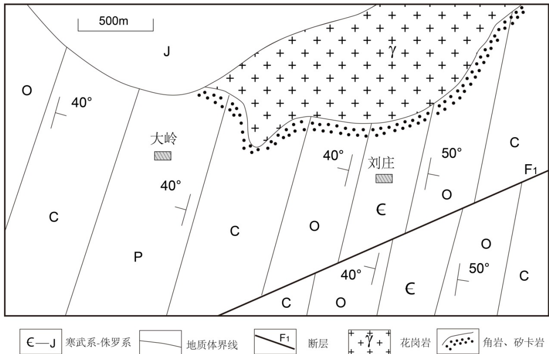
刘庄-大岭地区地质简图
